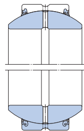
GEZH .. ES-2RS GEZH .. ES-2LS
